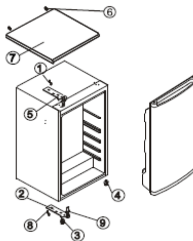
Fig. 2 Dörren öppnas från höger sida
